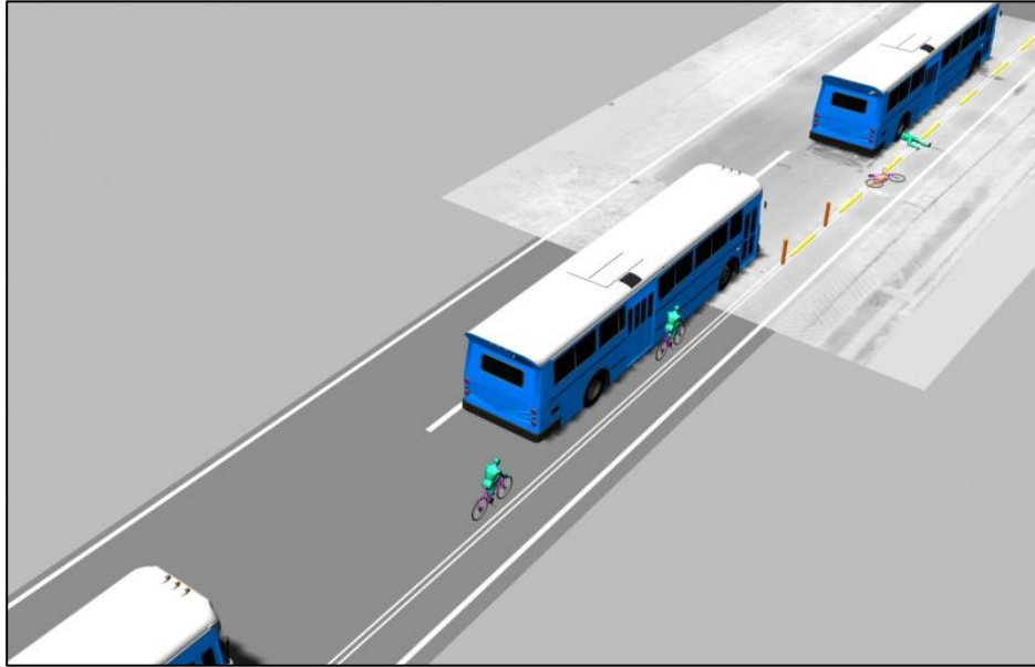
Figura N° 22: Resultado de la simulación por PC-Crash®, con referencia de escaneo.
