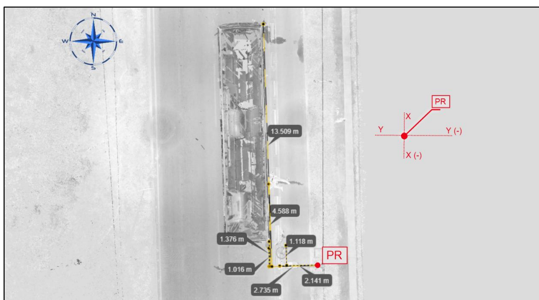
Figura N°16: Mediciones tomadas durante la navegación en el entorno escaneado en la Copia del Documento N° 5]: Copia de archivo de Escaneo con Faro Focus 3D.
