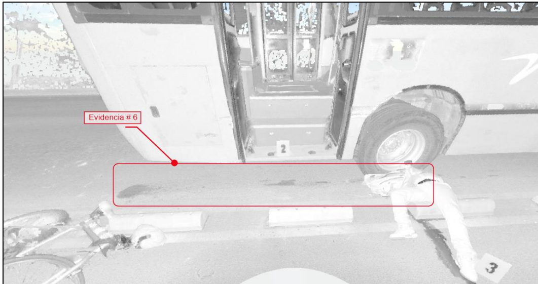
Figura N° 21: Marca de arrastre orgánico. Captura de navegación vista de Oriente a Occidente, del archivo SCENE 2go . Documento N° 5]: Copia de archivo de Escaneo con Faro Focus 3D).
