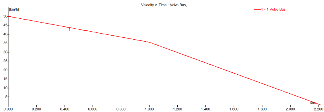
Figura N° 23: Gráficas de velocidad – tiempo para Vehículo #1: bus marca Volvo, línea B7R, placas VCS-572, obtenidos por la simulación con PC-Crash®.
