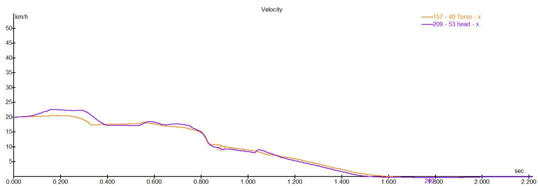
Figura N° 24: Gráficas de velocidad – tiempo para el torso y la cabeza de la víctima, obtenidos por la simulación con PC-Crash®.
