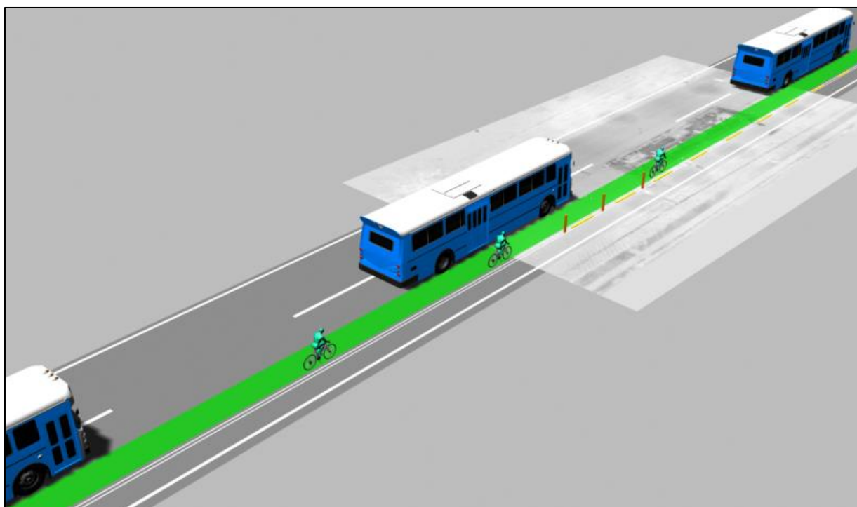
Figura N° 29: resultado de la simulación de evitabilidad de la colisión.
