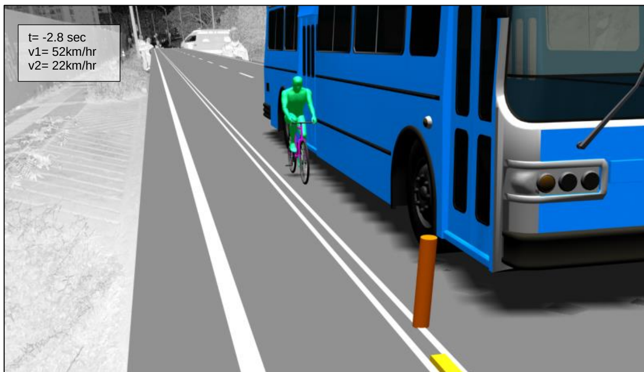
Figura N° 26: vista sobre escaneo del vehículo #1: bus marca Volvo, línea B7R, placa VCS-572, colisionado con su lateral derecho sobre el vehículo #2: bicicleta color morado, marco N° 11015.
