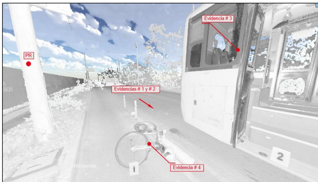
Figura N° 15: captura de navegación vista de Norte a Sur, del archivo SCENE 2go. Documento N° 5]: Copia de archivo de Escaneo con Faro Focus 3D).
