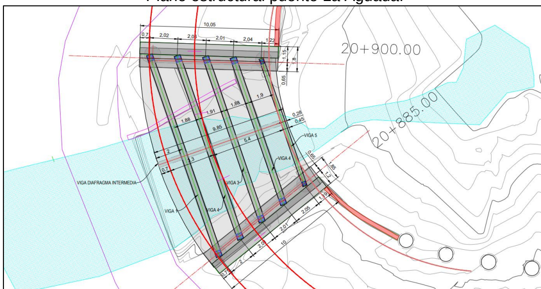
Imagen 3. Plano estructural puente La Aguada.
