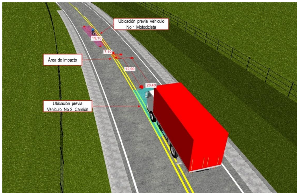
Imagen No.38: En esta imagen, se observa el área de ubicación relativa entre los vehículos involucrados 1,2s y 1,5s antes del área de impacto. Elaborada en el software Trimble Forensic Reveal
