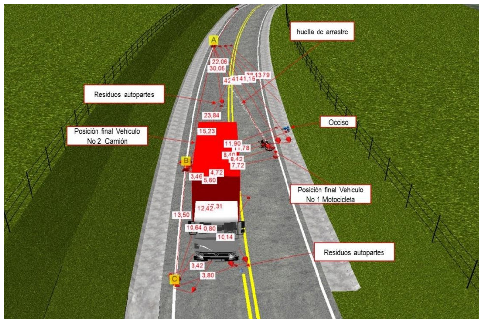
Imagen No. 26: En esta imagen vista en 3D se observa la elaboración a escala del evento en el software Trimble Forensic Reveal.
