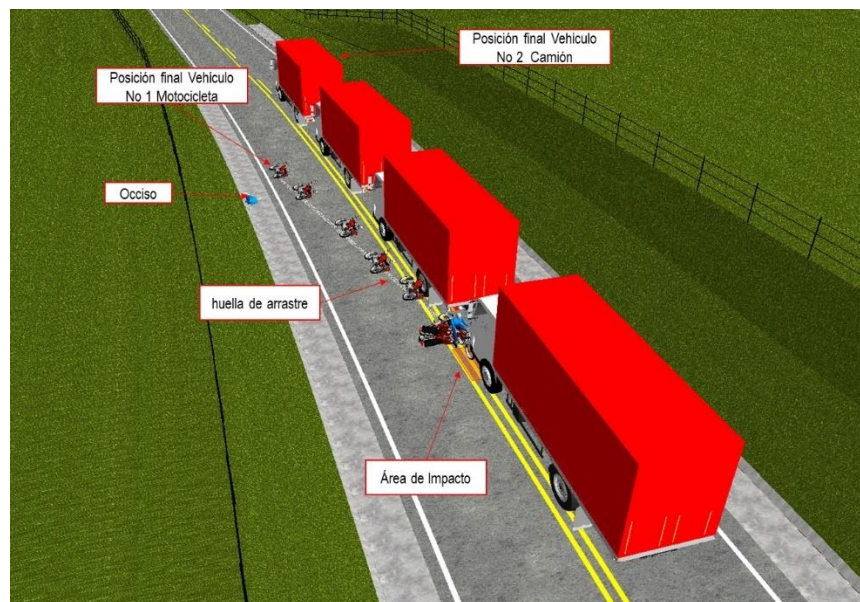
Imagen No. 36: En esta imagen en 3D, se observa la secuencia del accidente, nótese el sentido de desplazamiento de los vehículos, el área de impacto de color naranja. Elaborada en el software Trimble Forensic Reveal.
