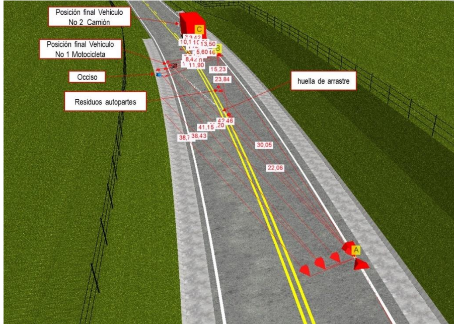
Imagen No. 27: En esta imagen vista en 3D se observa la elaboración a escala del evento en el software Trimble Forensic Reveal.
