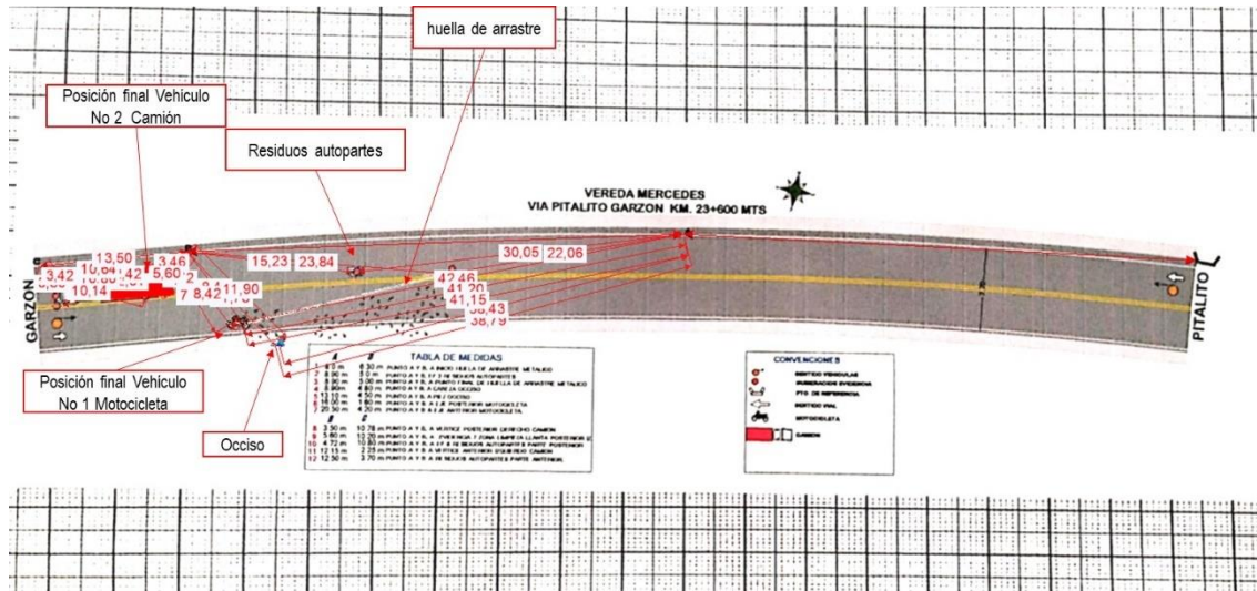
Imagen No. 23: En esta imagen vista en planta se observa la elaboración a escala del evento en el software Trimble Forensic Reveal.
