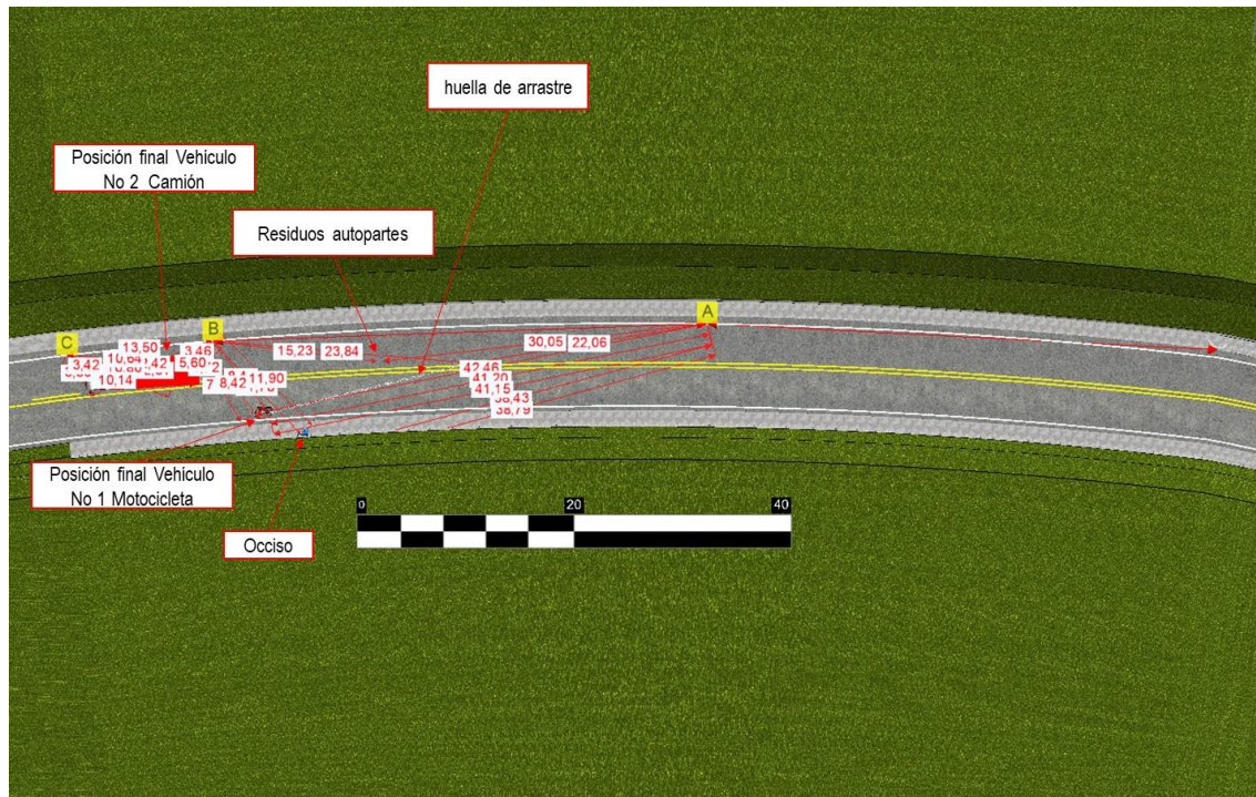
Imagen No. 24: En esta imagen vista en 3D se observa la elaboración a escala del evento en el software Trimble Forensic Reveal.
