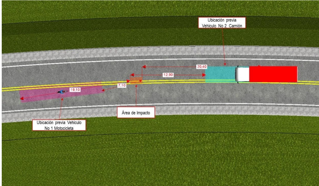
Imagen No.37: En esta imagen, se observa el área de ubicación relativa entre los vehículos involucrados 1,2s y 1,5s antes del área de impacto. Elaborada en el software Trimble Forensic Reveal
