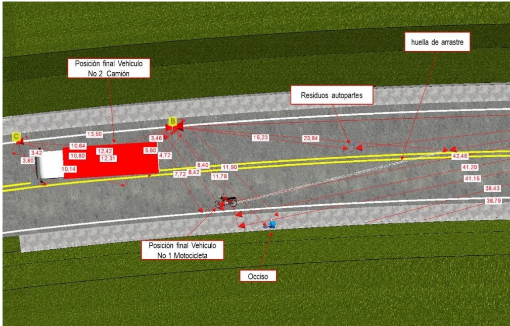
Imagen No. 25: En esta imagen vista en 3D se observa la elaboración a escala del evento en el software Trimble Forensic Reveal.
