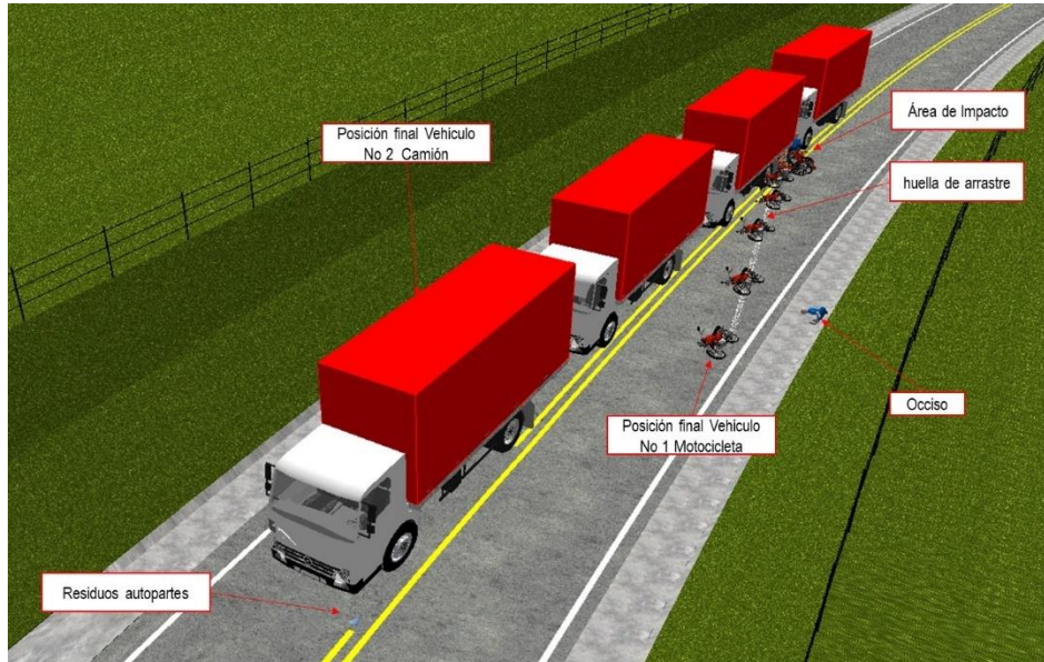
Imagen No. 35: En esta imagen, vista en planta se observa la secuencia del accidente, nótese el sentido de desplazamiento de los vehículos, el área de impacto de color naranja, y sus desplazamientos hasta sus posiciones finales. Elaborada en el software Trimble Forensic Reveal
