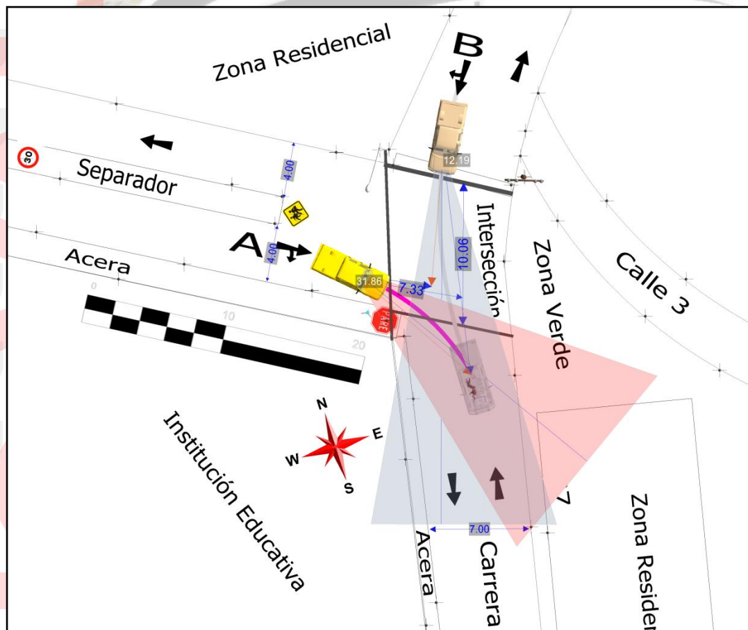
Ilustración 35. Fuente UIFCP: vista en modelo 2D de la trayectoria de vehículo (1) en sendero pre impacto y post impacto según Intersección tipo (Y)
