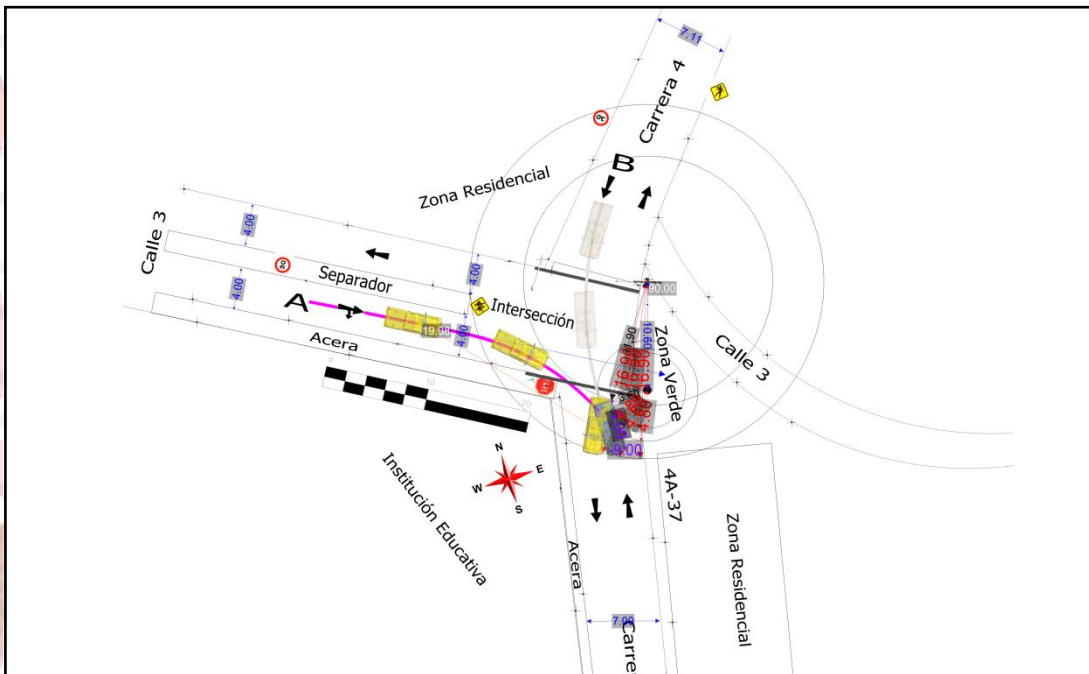
Ilustración 25. Fuente UIFCP, representación grafica 2D general - análisis de la trayectoria del vehículo (1) sobre la intercepción tipo (Y) En sendero pre-impacto según información técnica observada.
