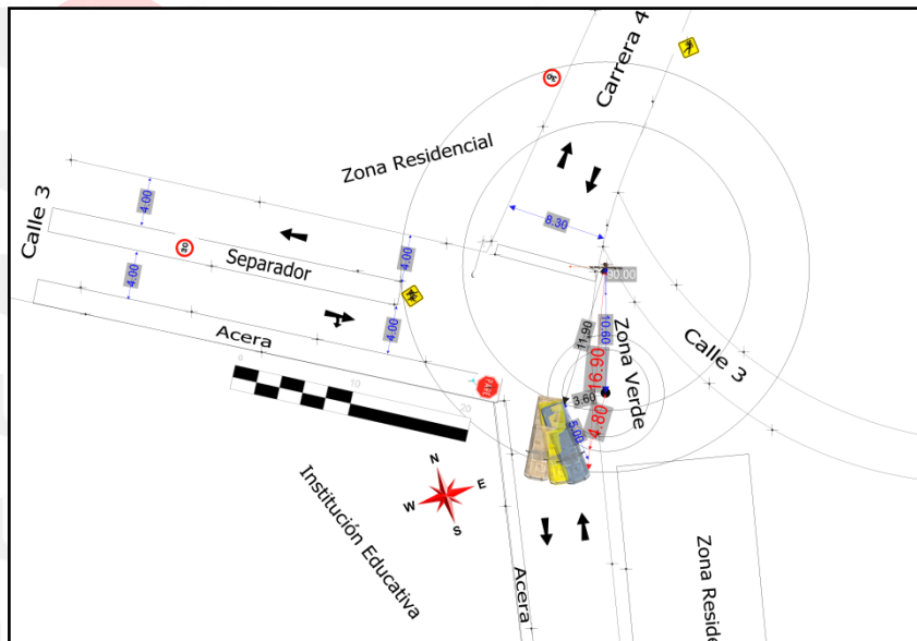
Ilustración 17. Fuente UIFCP, Representación gráfica bidimensional (2D), replanteo de información de EF/EMP Plano General
