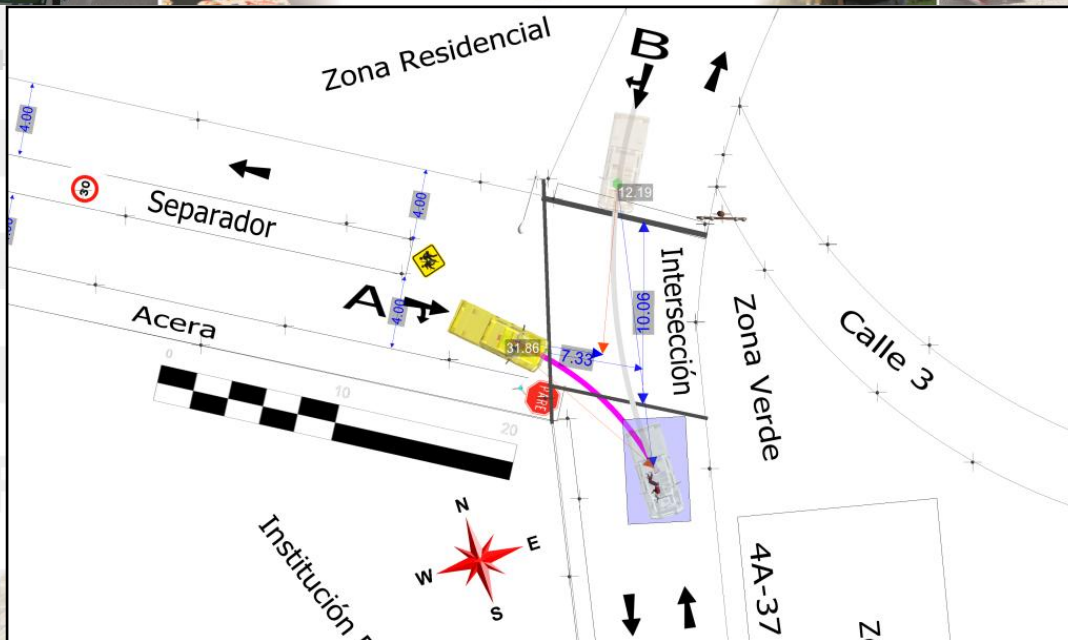
Ilustración 33. Fuente UFCP: representación grafica 2D general - análisis de la trayectoria del vehículo (1) sobre la intersección tipo (Y) Vs PF (víctima) Trayectoria A: recorrido superior a 7.33m intersección tipo (Y) → giro entre 0^\circ \geq 31.86^\circ Trayectoria B: recorrido superior a 10.06m intersección tipo (Y) → giro entre 0^\circ \geq 12.19^\circ En sendero pre-impacto según información técnica observada. : Zona de conflicto
