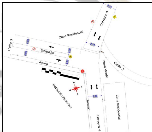
Ilustración 8. Fuente UFCP: Representación grafica bidimensional 2D; Replanteo de la información (EF y/o EMP) del dibujo topográfico del día de los hechos. Imagen a escala propia
