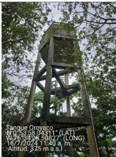
Imagen 80 Tanque Oroyaco.
