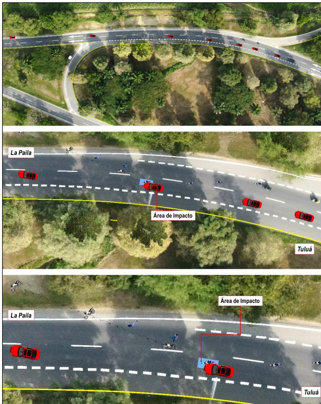
Imagen No. 24: En estas imágenes vista en planta 3D se observa la secuencia del accidente, nótese el sentido de desplazamiento de los vehículos, el área de impacto de color azul y sus desplazamientos hasta sus posiciones finales.
