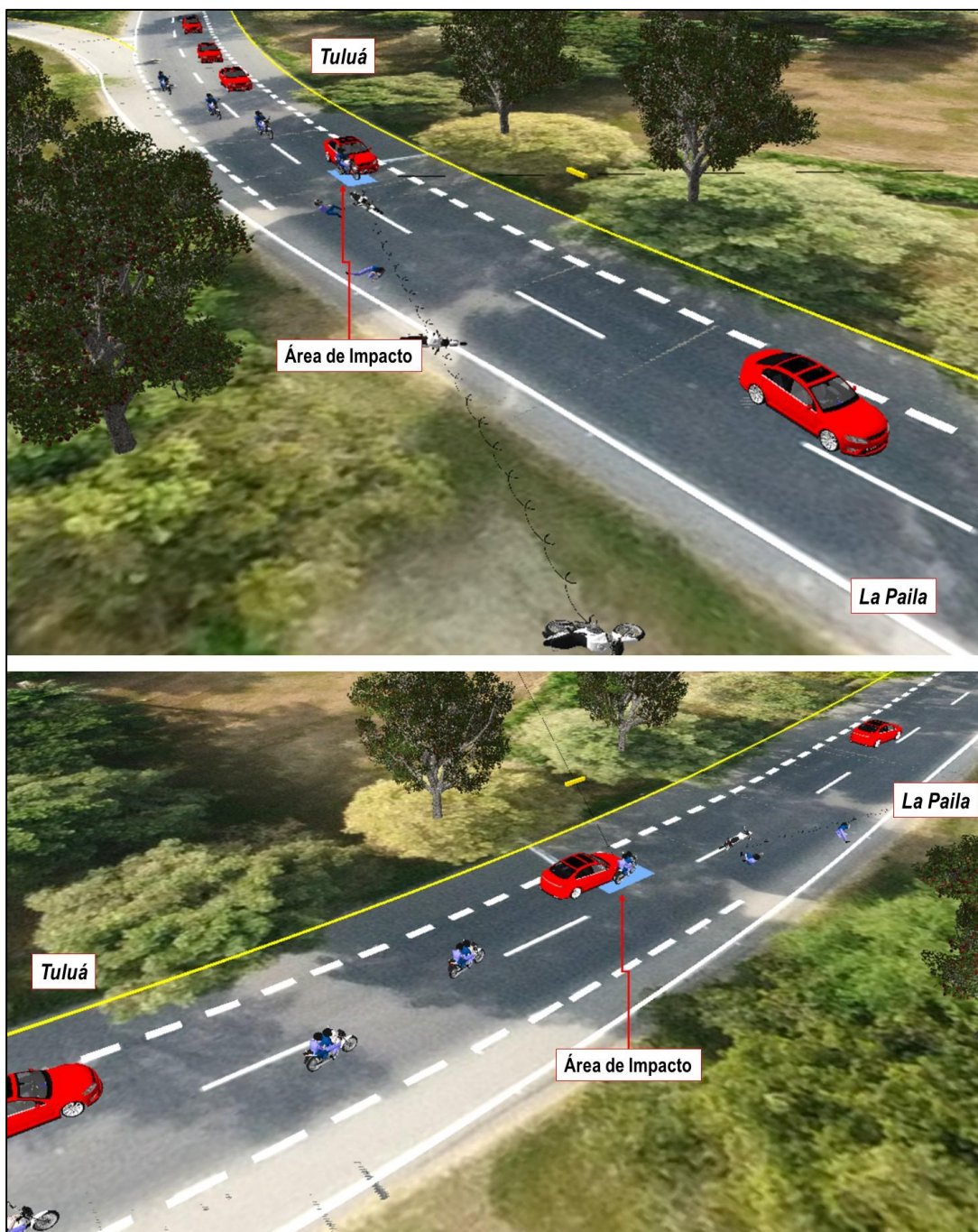
Imagen No. 25 En estas imágenes vista en perspectiva 3D se observa la secuencia del accidente, nótese el sentido de desplazamiento de los vehículos, el área de impacto de color azul y sus desplazamientos hasta sus posiciones finales.
