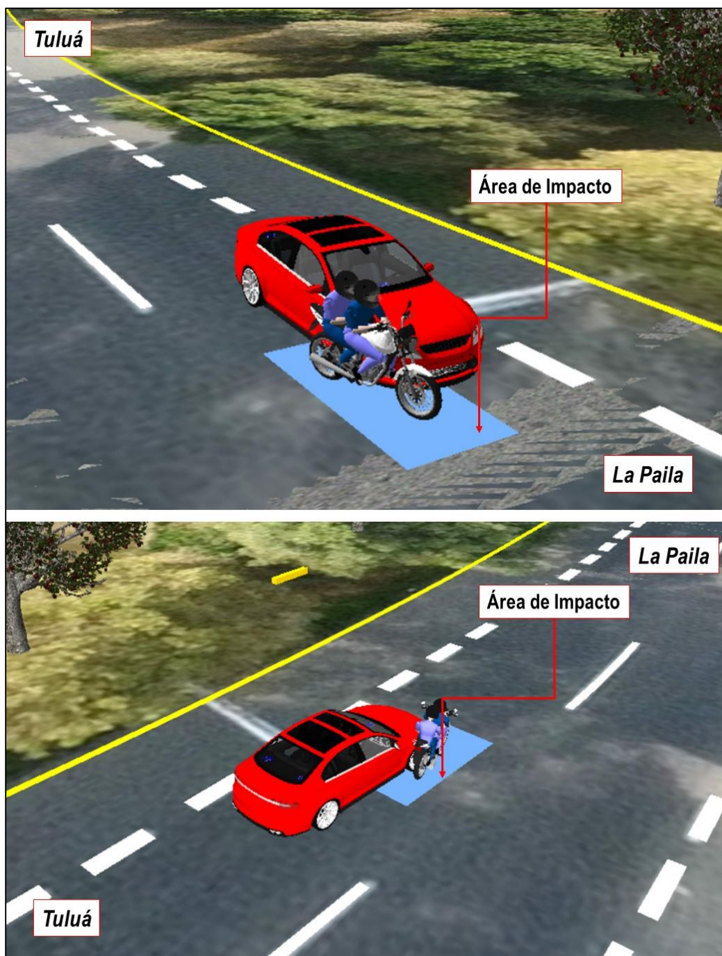
Imagen No.19: En esta imagen en perspectiva 3D se muestra la posición relativa de los involucrados al momento del impacto, y el área azul de colisión.
