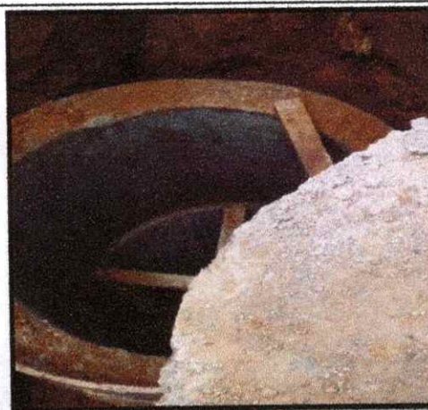
FOTOGRAFIA 4: CONSTRUCCION DE LA CAMARA DE INSPECCION N°17 DEL ALCANTARILLADO PLUVIAL
