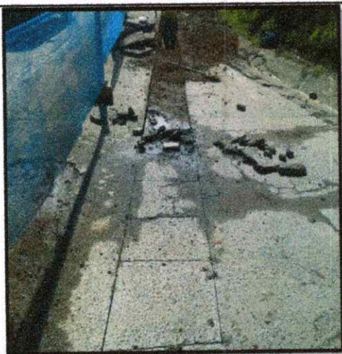
FOTOGRAFIA 1: DEMOLICION Y CORTE DE PAVIMENTO ASFALTICO PARA INSTALACION DE TUBERIA DE 6" DE LA RED DE DISTRIBUCION DE ACUEDUCTO
