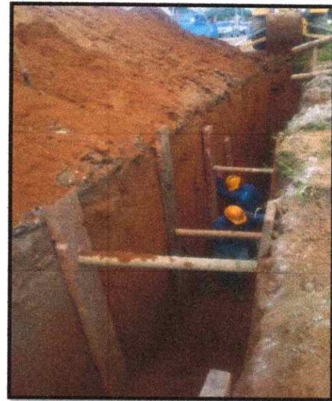
FOTOGRAFIA 6: ENTIBADO APUNTALADO EN EL TRAMO DESDE LA CAMARA 20 A LA CAMARA 19 DEL ALCANTARILLADO PLUVIAL
