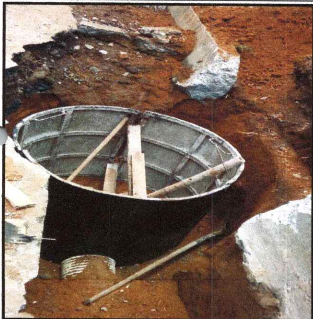
FOTOGRAFIA 7: INSTALACION DE FORMALETA PARA CONSTRUCCION LA CAMARA 11 DEL ALCANTARILLADO PLUVIAL
