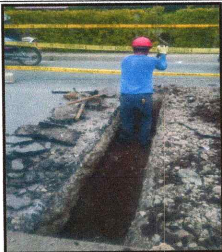
FOTOGRAFIA 1: EXCAVACION A MANO PARA INSTALACION DE TUBERIA DE 8" DE LA RED DE DISTRIBUCION DE ACUEDUCTO
