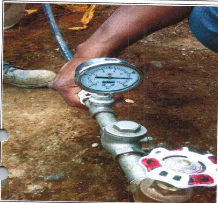
REALIZACION DE PRUEBA HIDROSTATICA RED DE ACUEDUCTO TRAMO I DESDE LA VARIANTE HASTA LA LICORERIA SAN DIEGO
