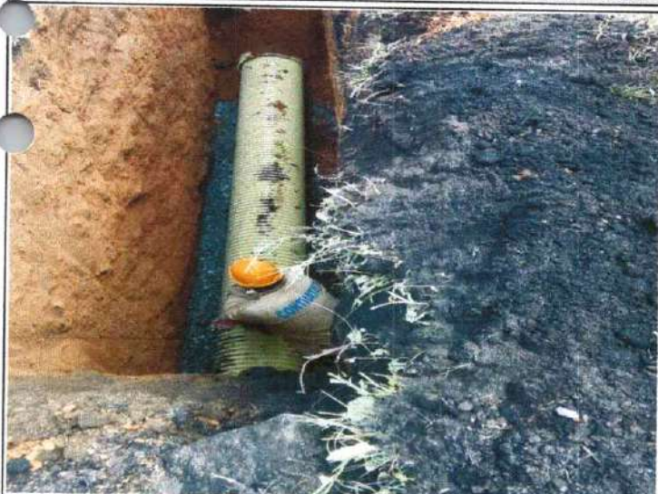
INSTALACION DE TUBERIA PARA ALCANTARILLADO SANITARIO DE 18"
