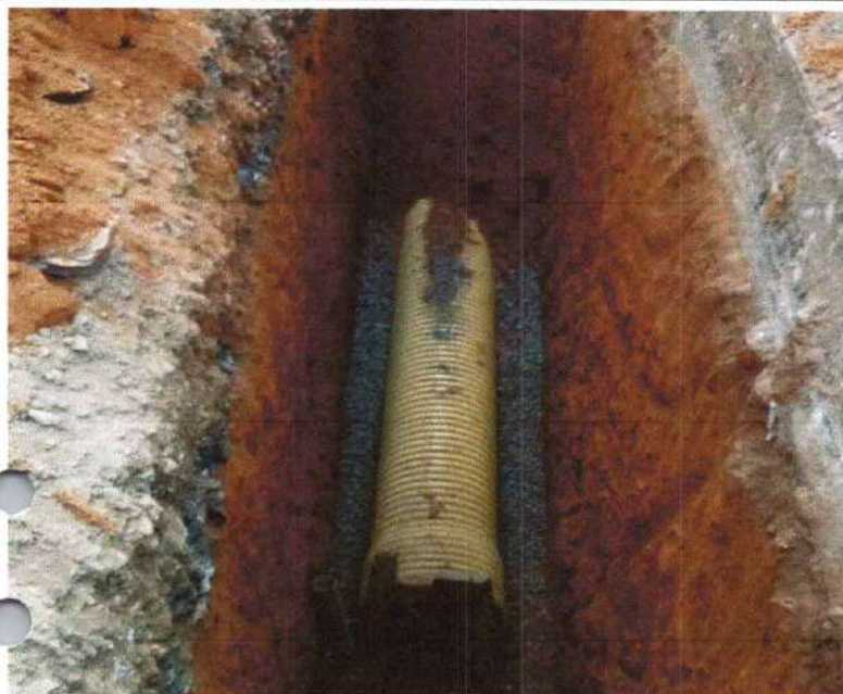
INSTALACION DE TUBERIA PLUVIAL TRAMO I DE 20"
