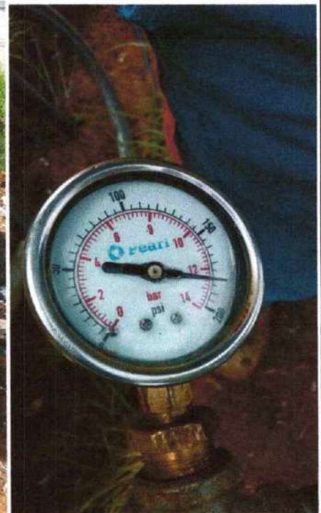
REALIZACION DE PRUEBA HIDROSTATICA RED DE ACUEDUCTO TRAMO I DESDE LA LICORERA SAN DIEGO HASTA LA PLACITA CAMPESINA
