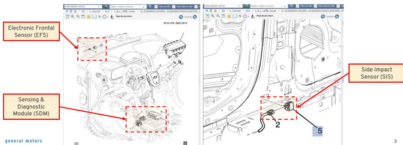
Imagen No. 8 Ubicación de sensores y airbag.
