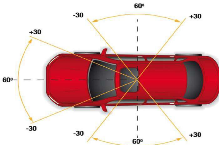
Imagen No. 10 Ángulos de activación frente al choque, depende la ubicación de los sensores y desaceleraciones. 3
