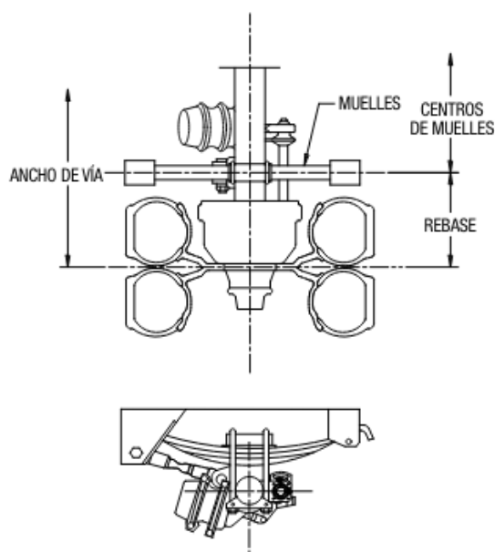
Imagen No. 7 Montaje suspensión rígida o ballestas
