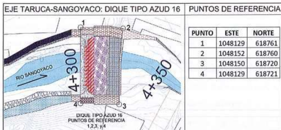
Dique tipo azud 16 (K4+310). Localización vista en planta
