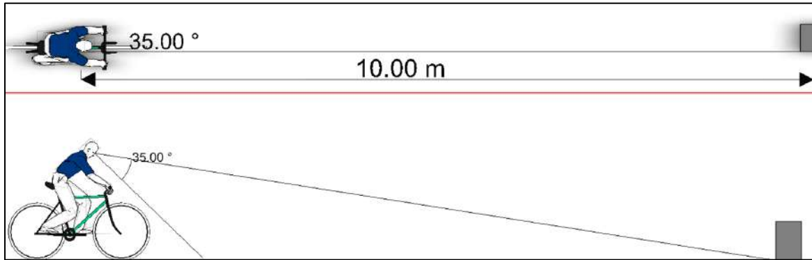
Imagen No.27: representación gráfica a escala en VC5 donde se ejemplifica el alcance del rango visual de la posición de un ciclista al inclinar la cabeza, contando un movimiento ocular hasta 35° (siendo casi el máximo los 25°).
