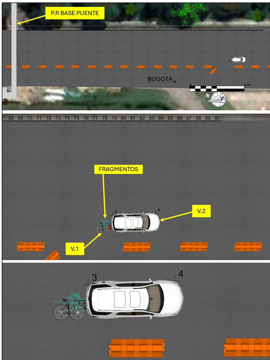
Imagen No.20: vista en planta de la construcción a escala en el software VirtualCrash5, del bosquejo elaborado para el evento por autoridad de tránsito.
