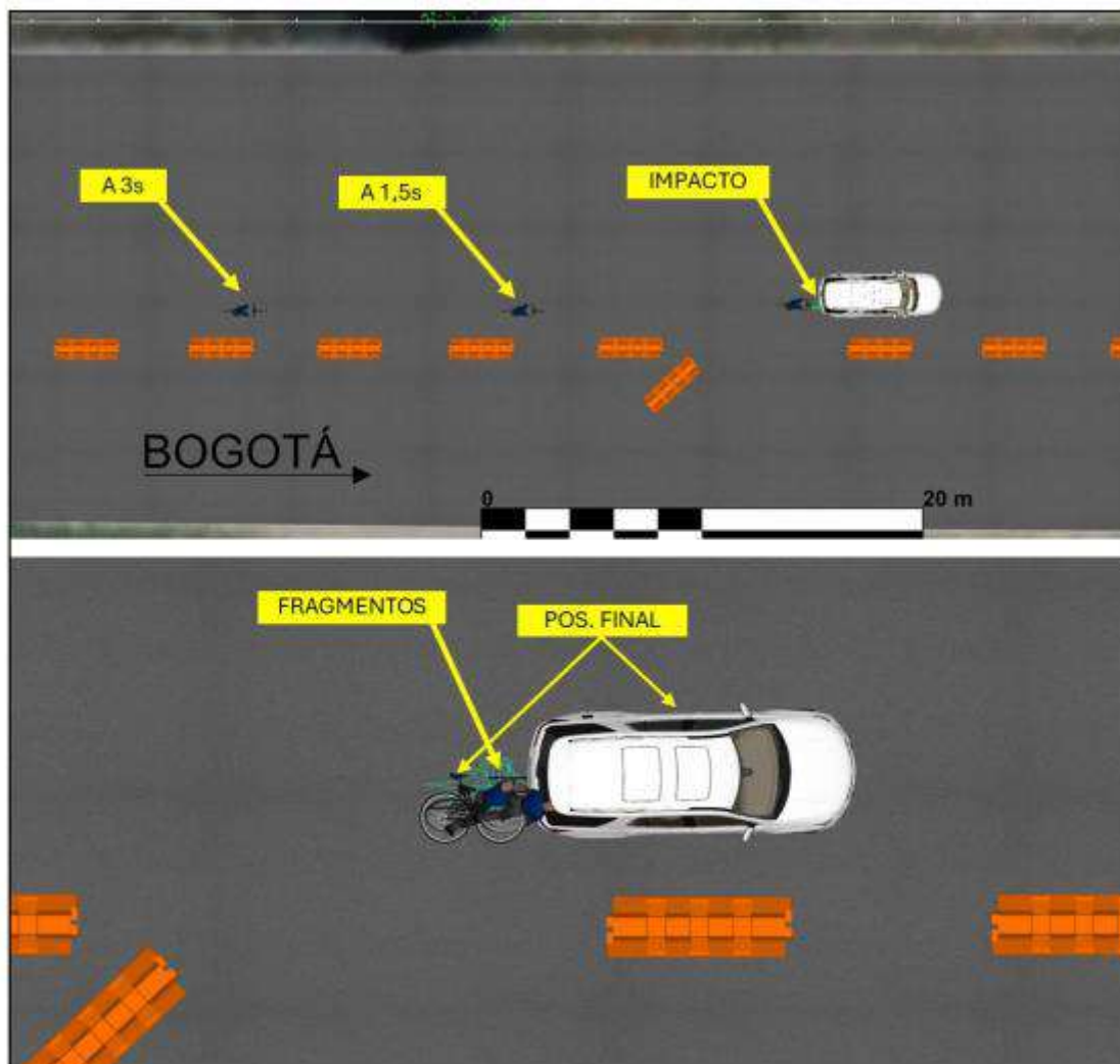
Imagen No.24: Compuesta por vista en planta del software VC5 donde se representa la secuencia probable del evento basados en el análisis forense de la evidencia registrada y recopilada. Se indica la ruta probable de aproximación al impacto, el momento y lugar de impacto en correlación con las posiciones finales y vestigios identificados.
