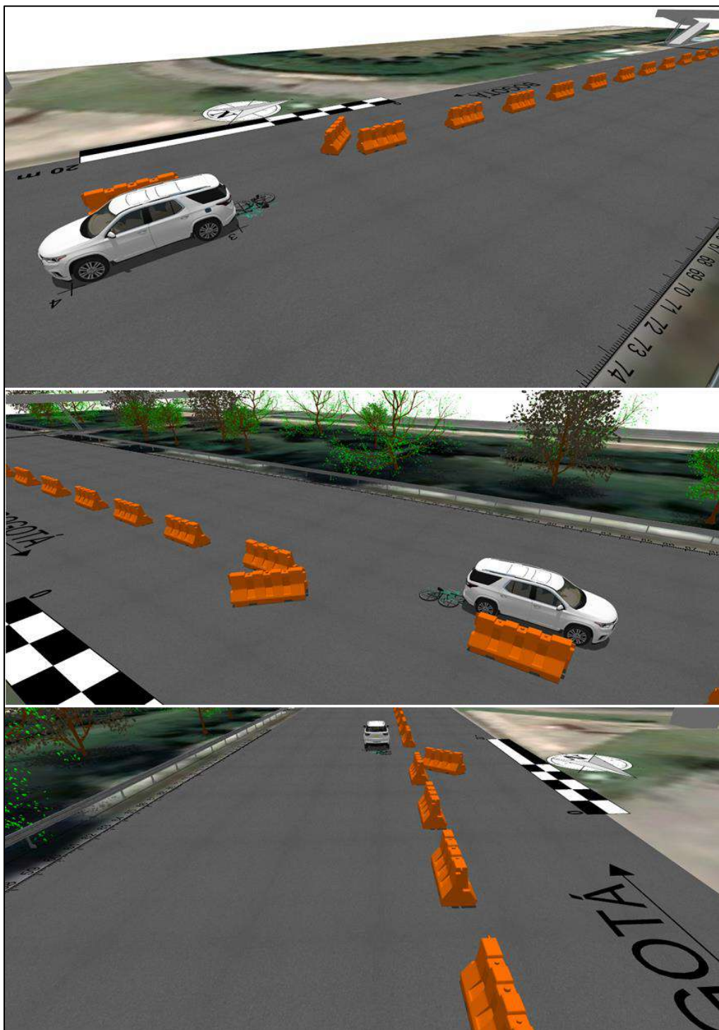
Imagen No.21: vista en 3D de la escena elaborada en el software VirtualCrash5.
