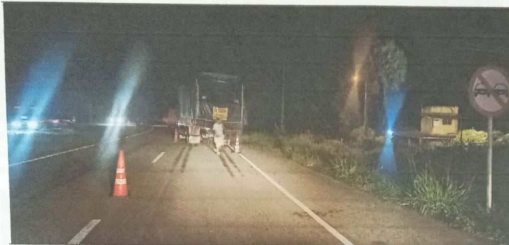
FOTOGRAFIA N° 01. PANORAMICA: SE OBSERVA EL LUGAR DE LOS HECHOS, UNA VIA PUBLICA ASFALTA, UNA CALZADA DOS CARRILES, UN SENTIDO VEHICULAR CON SEÑALIZACION HORIZONTAL, TALES COMO LINEA BLANCA DE BORDE Y SEÑALIZACION VERTICAL DE PROHIBIDO ADELANTAR.
