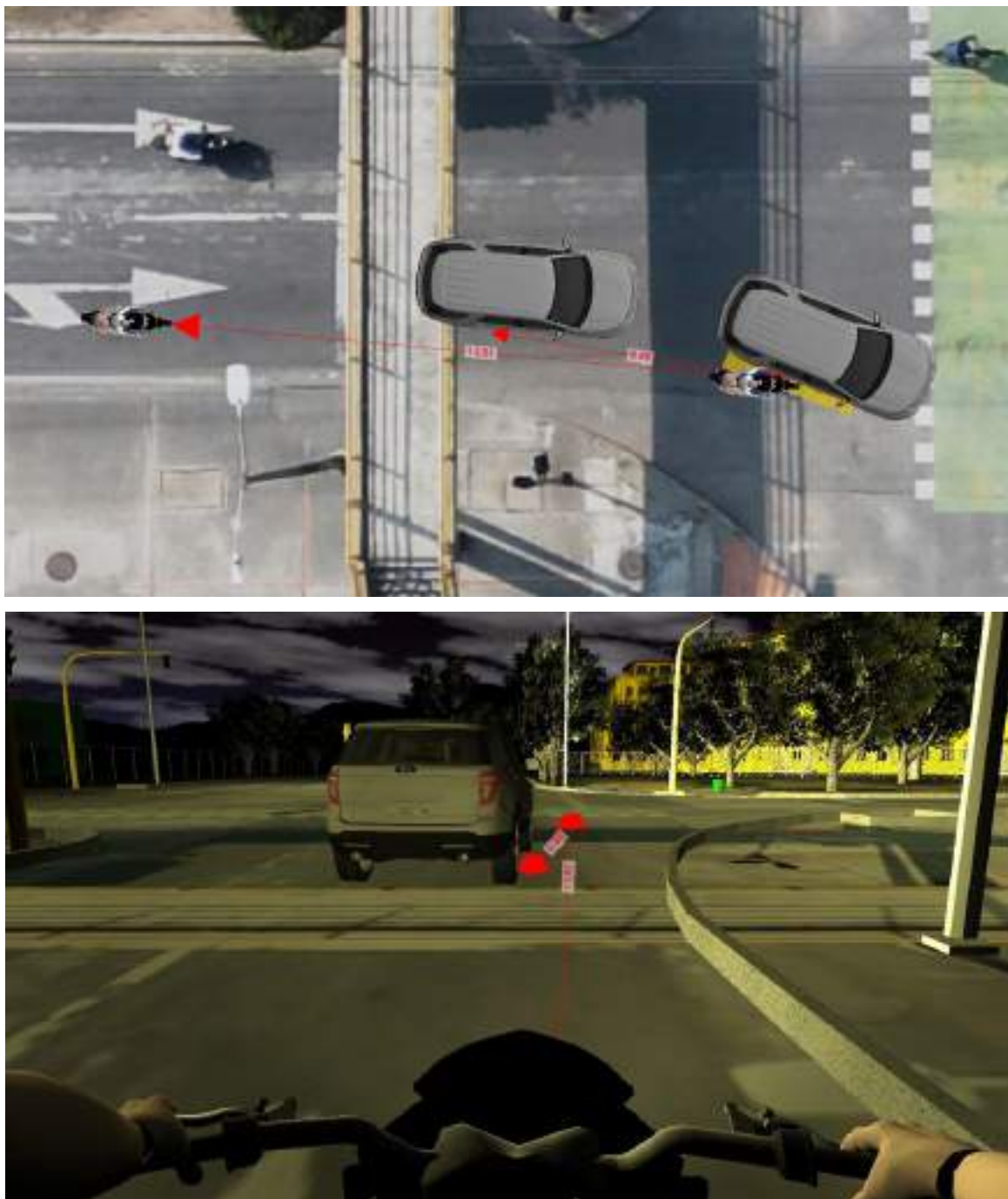
Imagen No. 54: En estas imágenes, vista en planta y 3D se aprecia la ubicación de los vehículos 1 s antes del impacto si sus velocidades son constantes y la visibilidad del conductor de la motocicleta. Elaboración a escala en el software Trimble Forensics Reveal.
