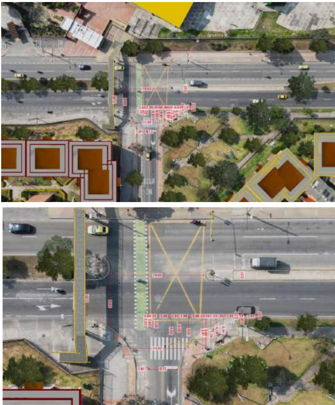
Imagen No. 43: En estas imágenes, vista en planta se observan las evidencias con base en las fotografías del día de los hechos. Elaboración a escala en el software Trimble Forensics Reveal.
