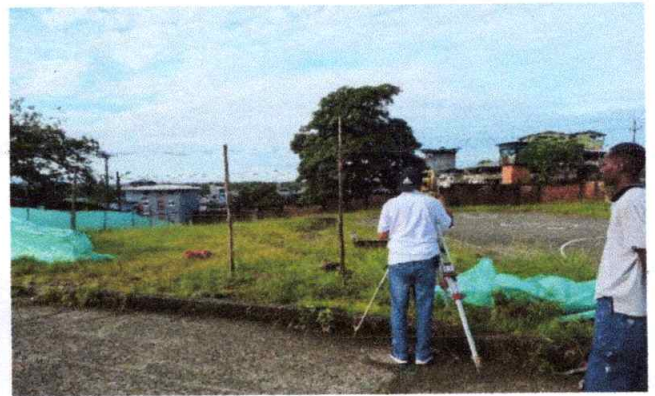
Foto 4: Localización y replanteo
