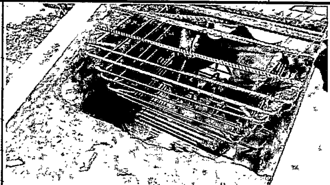
Foto 4. Colocación, armado y amarrado acero refuerzo + doble panilla para zapata en concreto.
