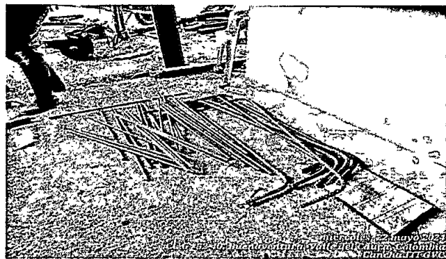
Foto 5: Corte y figurado de acero refuerzo.
