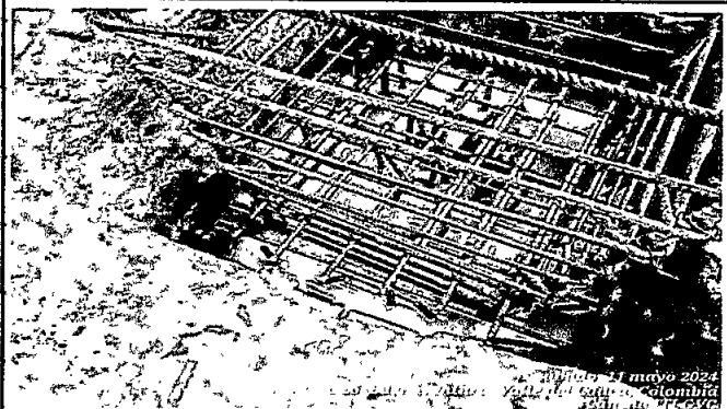
Foto 6. Colocación, armado y amarrado acero refuerzo + doble panilla para zapata en concreto.
