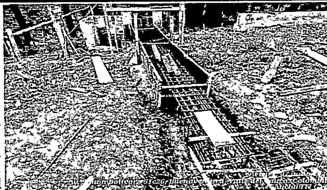
Foto 4: Encofrado de viga cimentación con formaleta metálica y en madera
