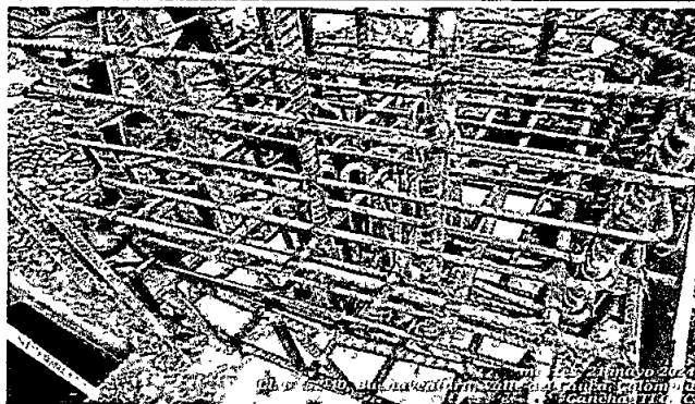
Foto 1: Colocación, armado y amarrado acero refuerzo + doble parrilla en zapatas y pedestales en concreto.
