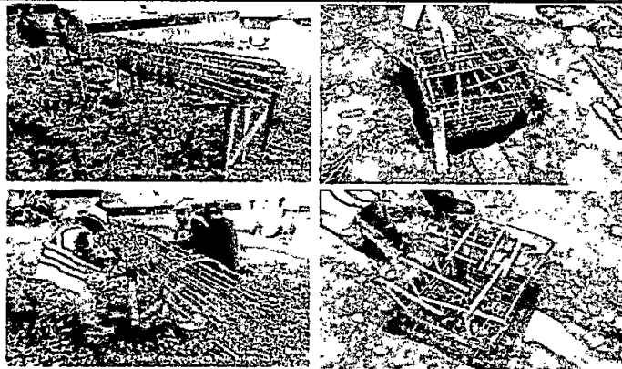
Foto 5: Corte, figurado y armado de estructura acero refuerzo para pilotes y pedestales
