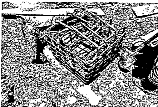
Foto 3: Colocación y armado acero refuerzo flejado para pedestal en concreto.
