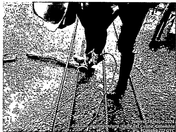
Corte y figurado de acero refuerzo para zapatas y pedestales en concreto.
