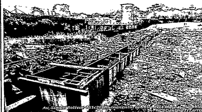
Foto 5: Encofrado de pedestales en madera
