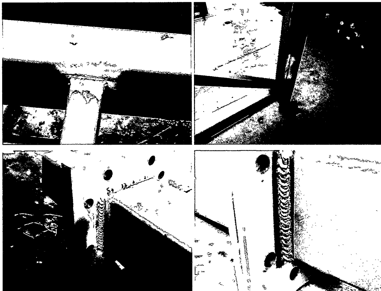
Fotografía 9-12. Inspección por líquidos penetrantes
