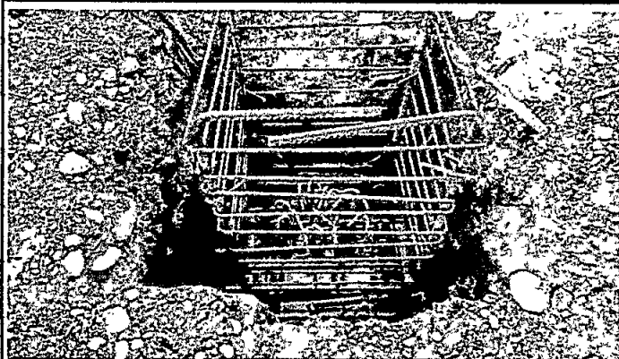
Foto 3: Colocación y armado acero refuerzo flejado para pedestal en concreto.
