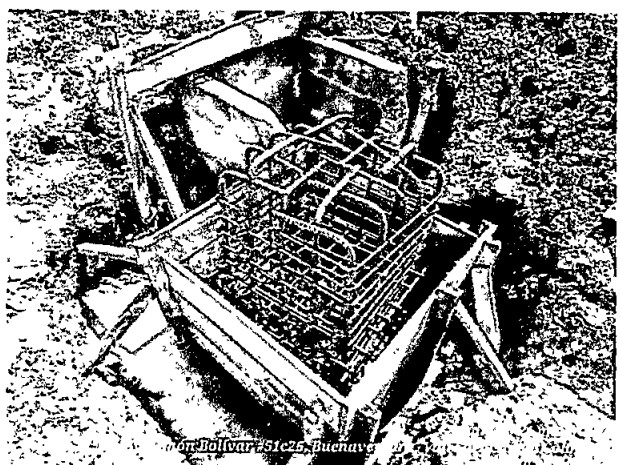
Armado y colocación en sitio de estructura acero refuerzo para zapatas y pedestales en concreto.
