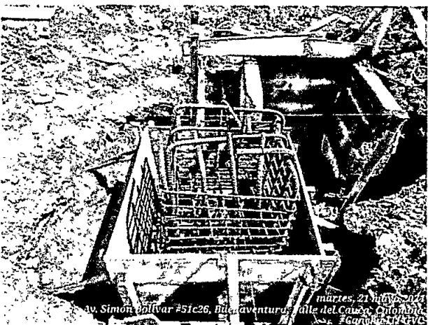
Carpintería en madera para encofrado de pedestales.
