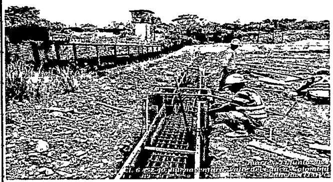
Foto 2: Encofrado de viga de concreto con formateo metálico y en madera.
