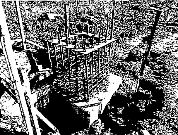
Colocación y/o ubicación de guías de las platinas para estructura metálica de la cubierta.
