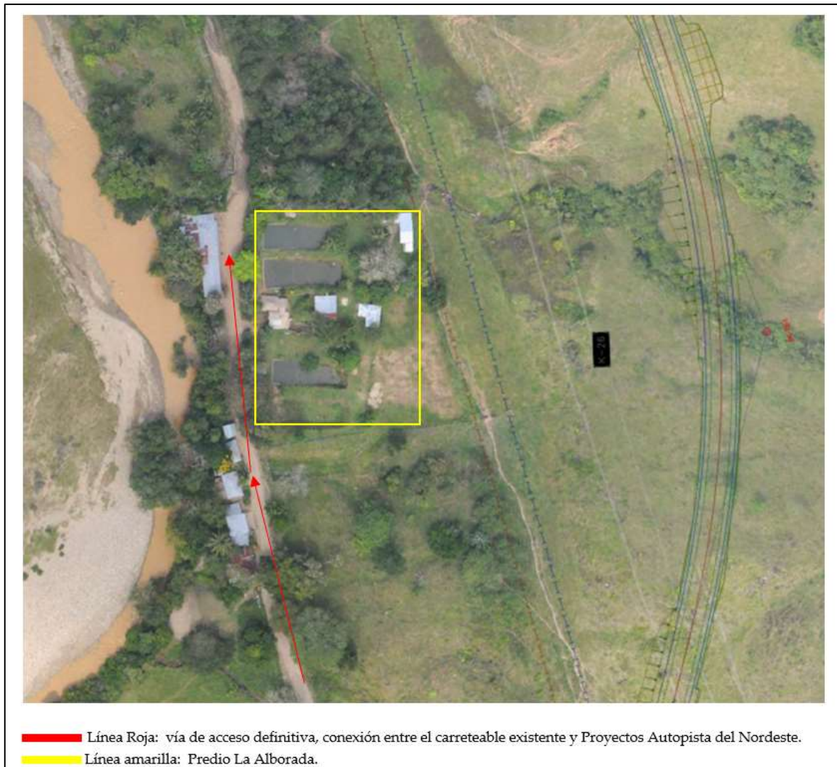
Imagen 4. Vía de acceso definitiva, conexión entre el carreteable existente y Proyectos Autopista del Nordeste.
