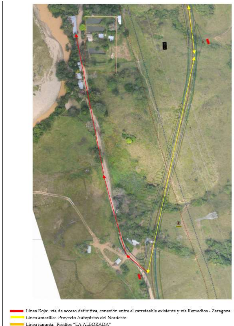
Imagen 3. Vía de acceso definitiva, conexión entre el carreteable existente y vía Remedios - Zaragoza
