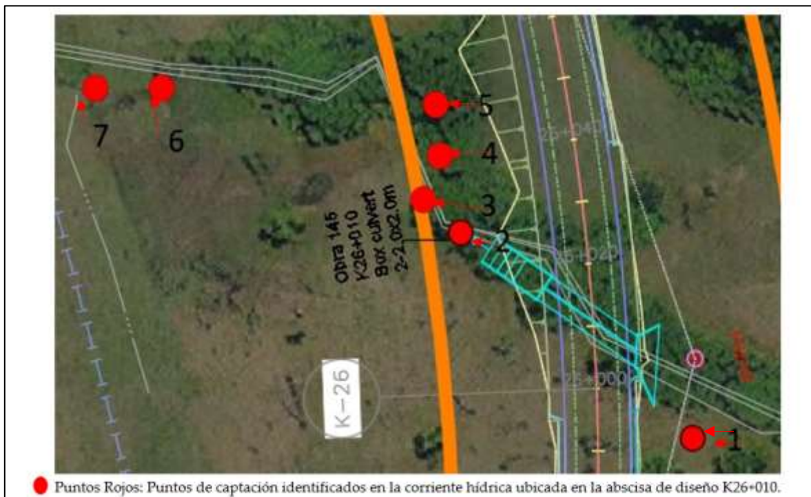
Imagen 5. Puntos de captación identificados en la fuente hídrica (K26+010)
