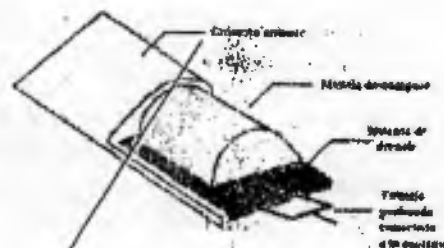
Figura 1.1.2. Sistema de tratamiento propuesto en la Fase 2 de la planta de biorremediación
