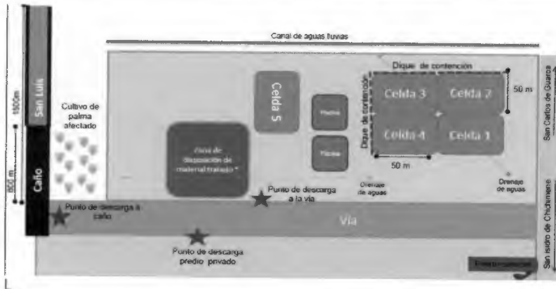
Figura 1. Diagrama del área de Bioremediación de la Planta de Tratamiento
