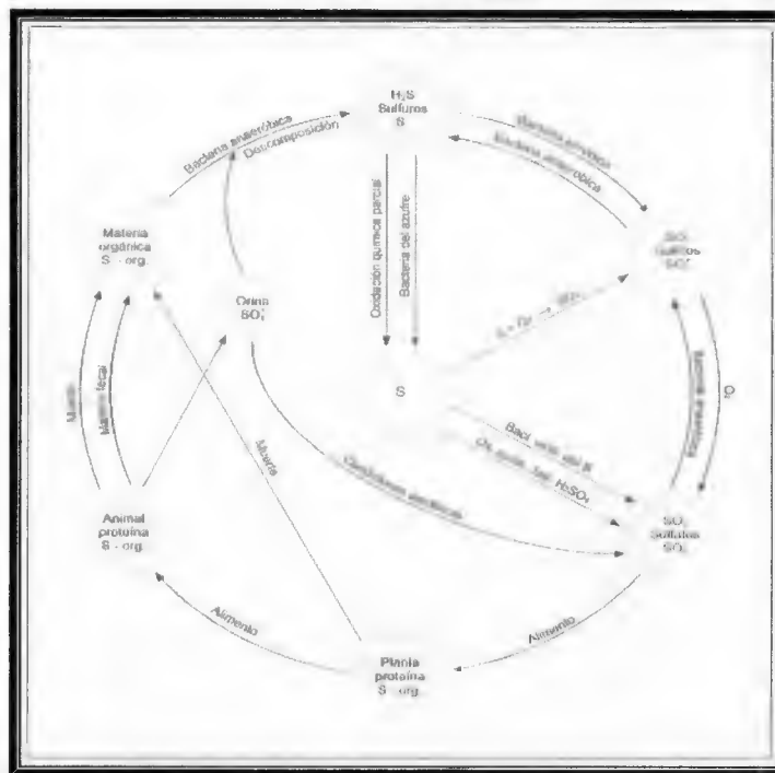
FIGURA 1. Ciclo del azufre
