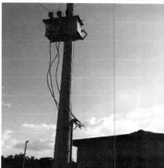
Equipos e instalaciones electromecánicas, vista general
